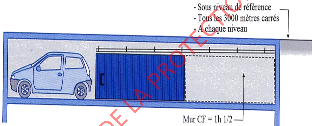
Figure 31 : Recouplement des parcs.
