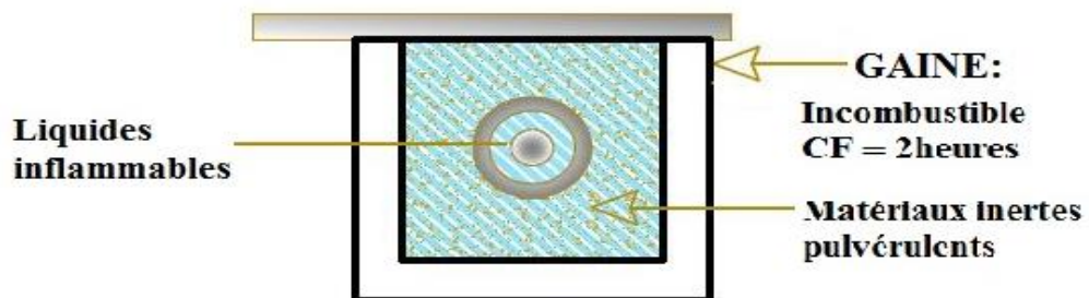
Figure 36 : Conduits de liquide inflammables.
