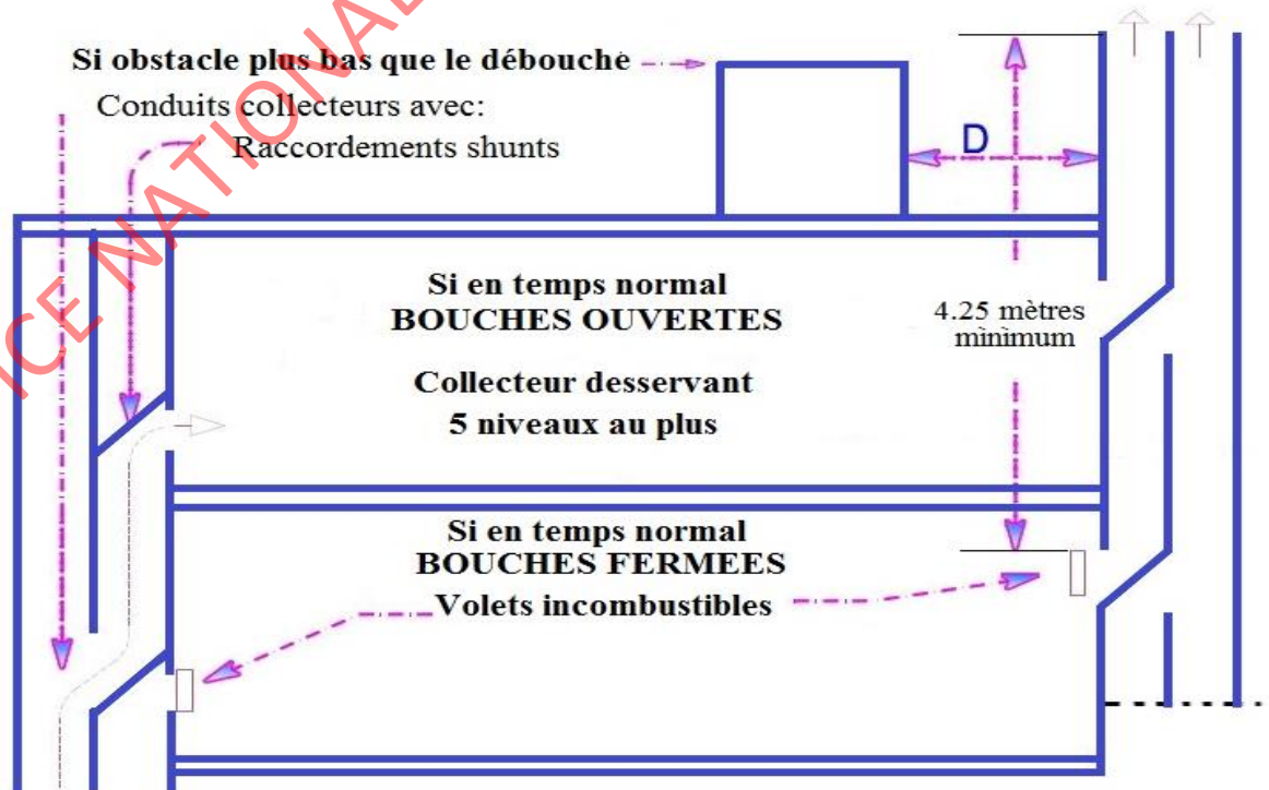
Figure 19 : Conduits collecteurs.
