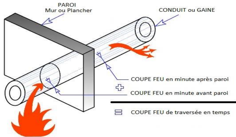
Figure 29 : Coupe feu de traversé.
