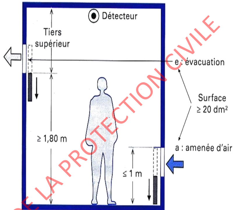
Figure 21 : Bouches de désenfumage.
