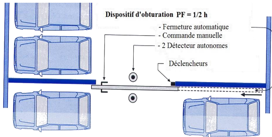
Figure 32 : Dispositif d'obturation.
