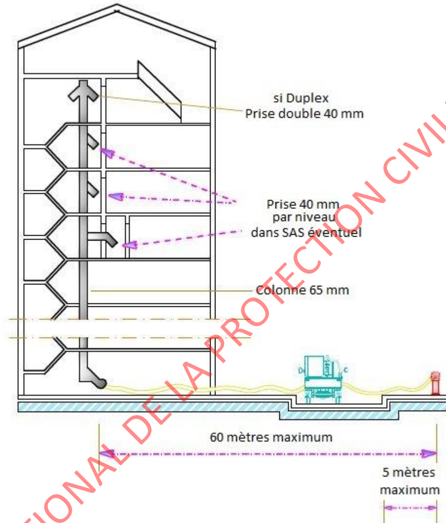
Figure 45 : Colonnes sèches.
