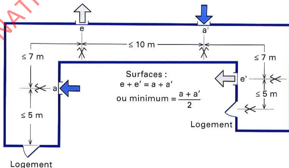
Figure 20 : Répartition et emplacement des bouches de désenfumage.
