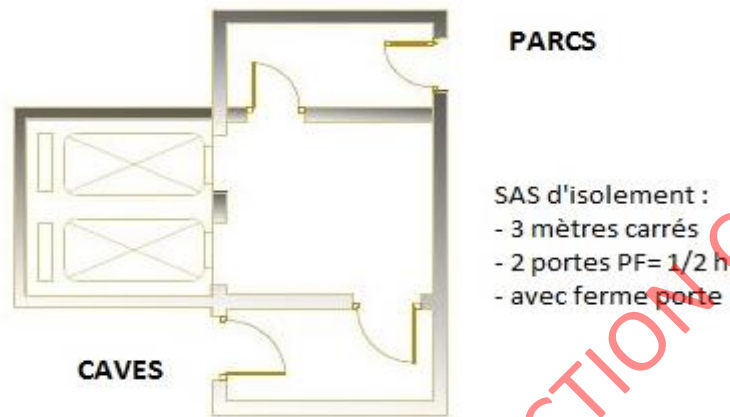
Figure 44 : SAS d'isolement avec parcs et caves.
