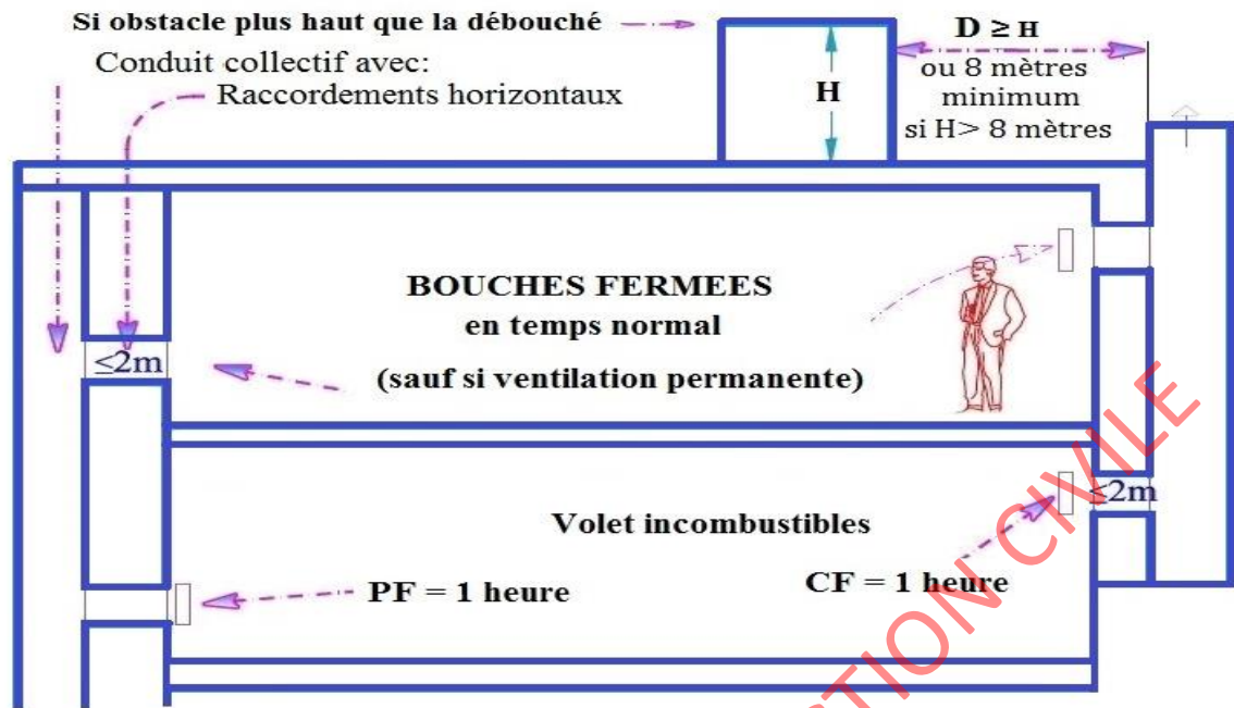
Figure 18 : Conduits collectifs.
