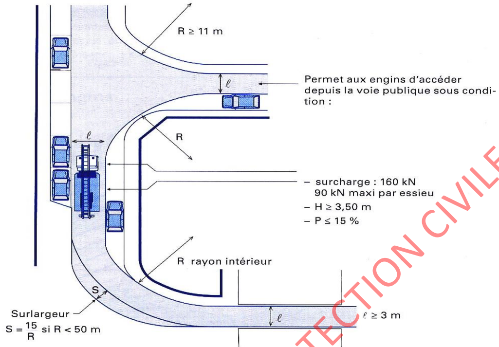
Figure 04 : Caractéristiques des voies engins.
