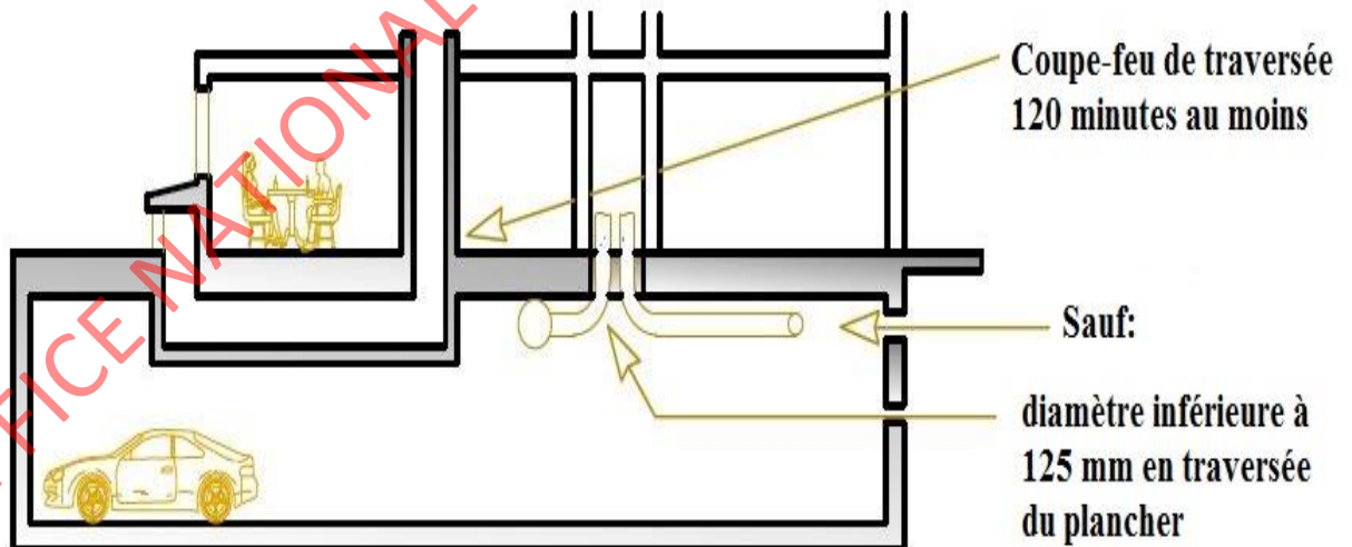
Figure 38 : Conduits de ventilation du parc.
