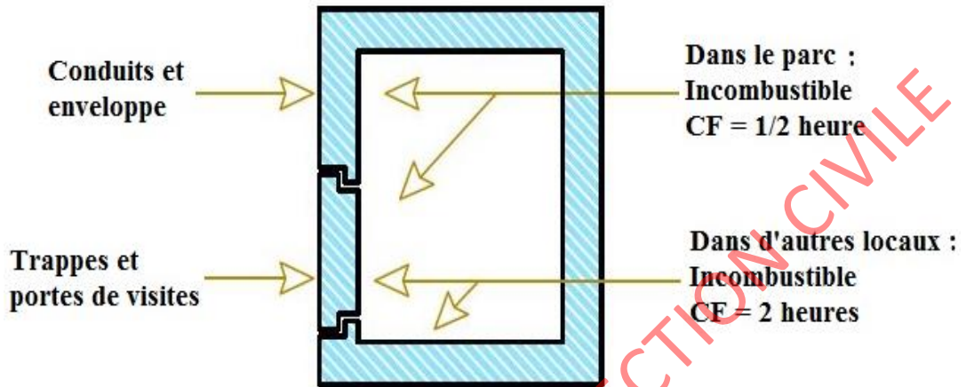
Figure 37 : Conduits de ventilation du parc.
