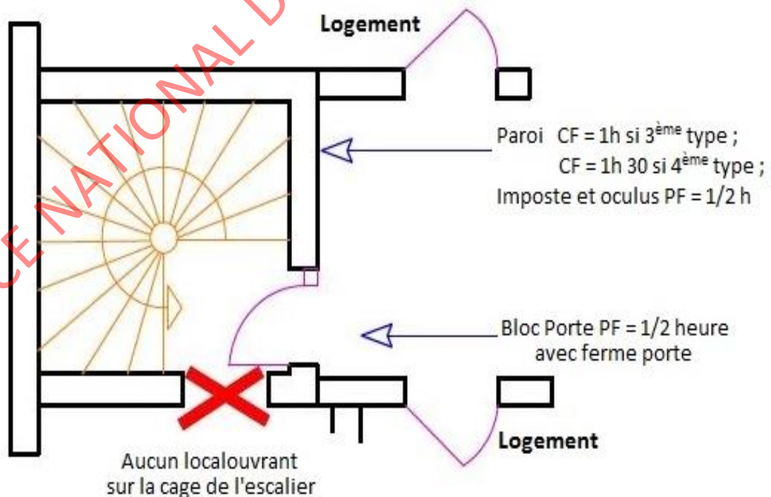
Figure 12 : Parois des escaliers non situées en façade.
