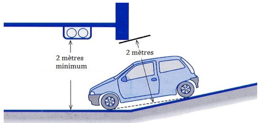
Figure 40 : Hauteur minimales des niveaux.
