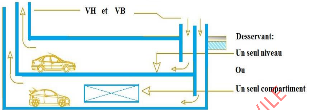
Figure 39 : Conduits de ventilation du parc.
