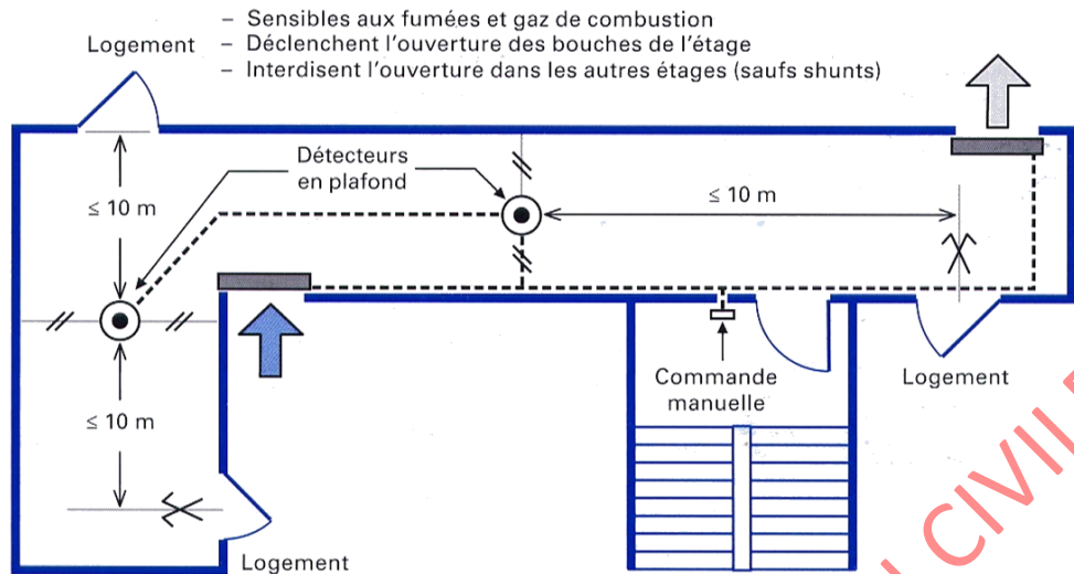
Figure 22 : DéTECTEURS.
