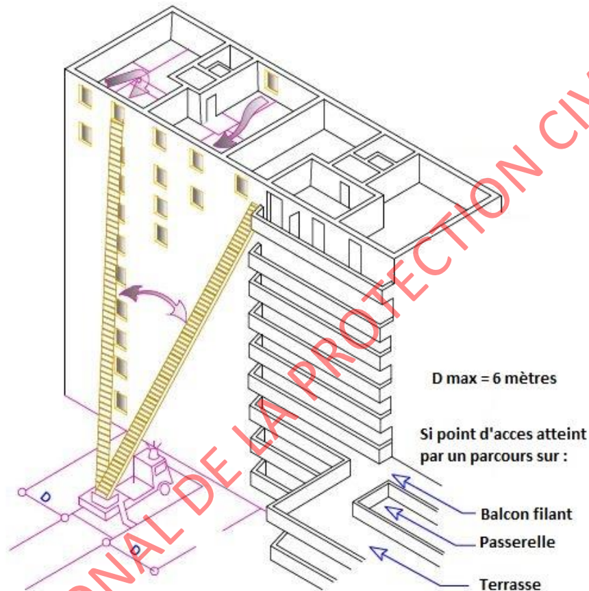
Figure 07 : Caractéristiques des voies échelles.
